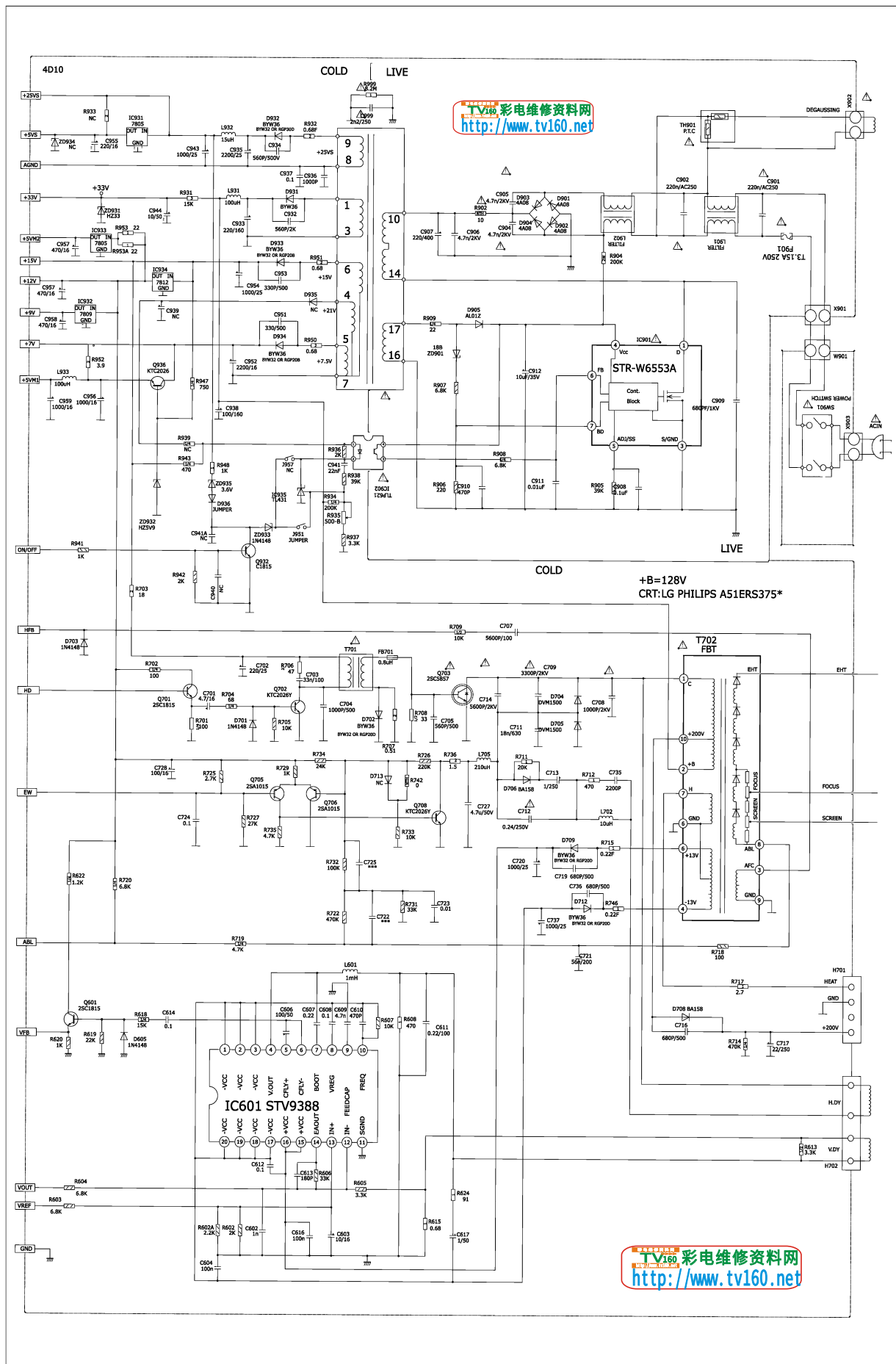
3D10主板原理图
