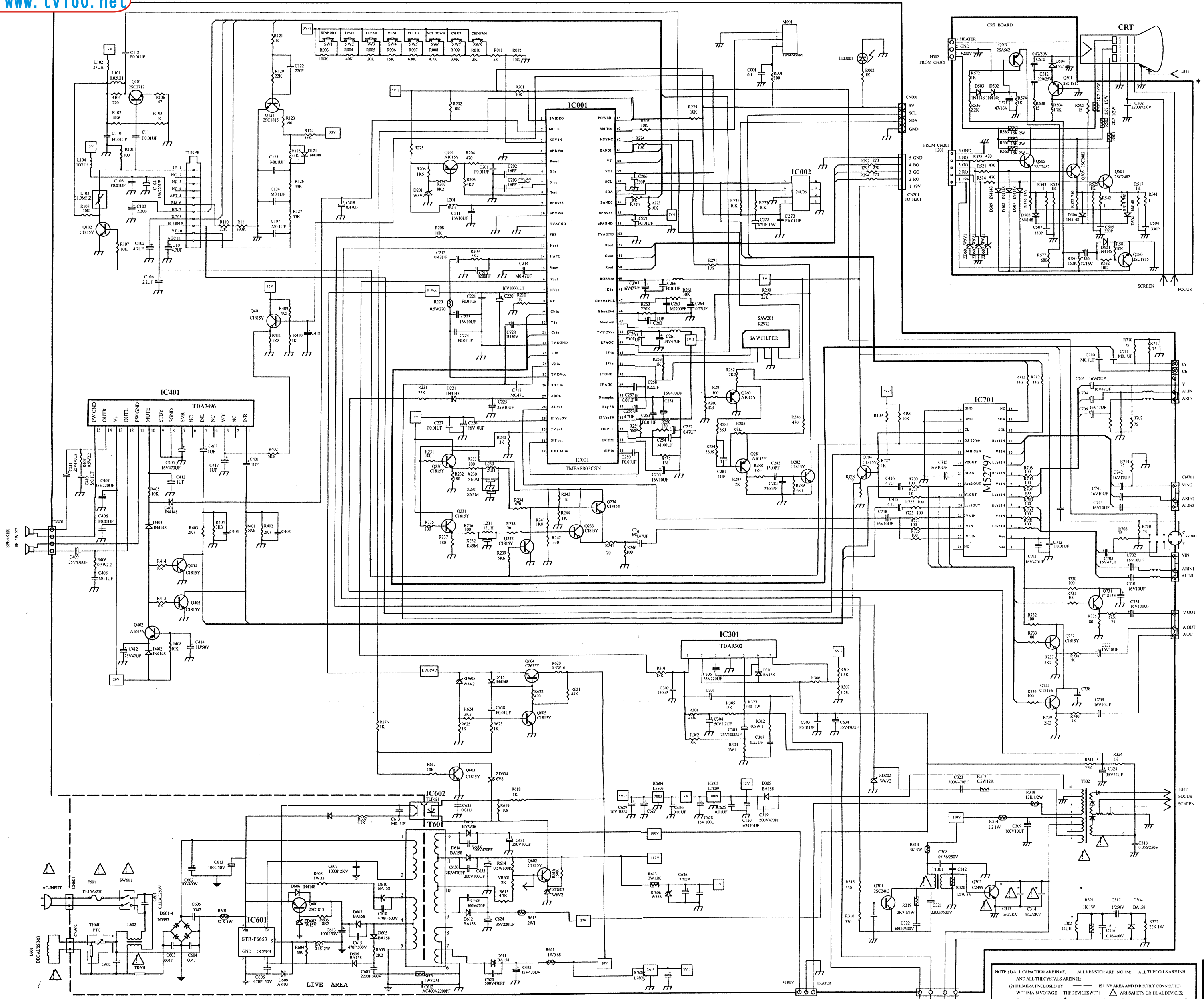
附录 3T30机芯电原理图
