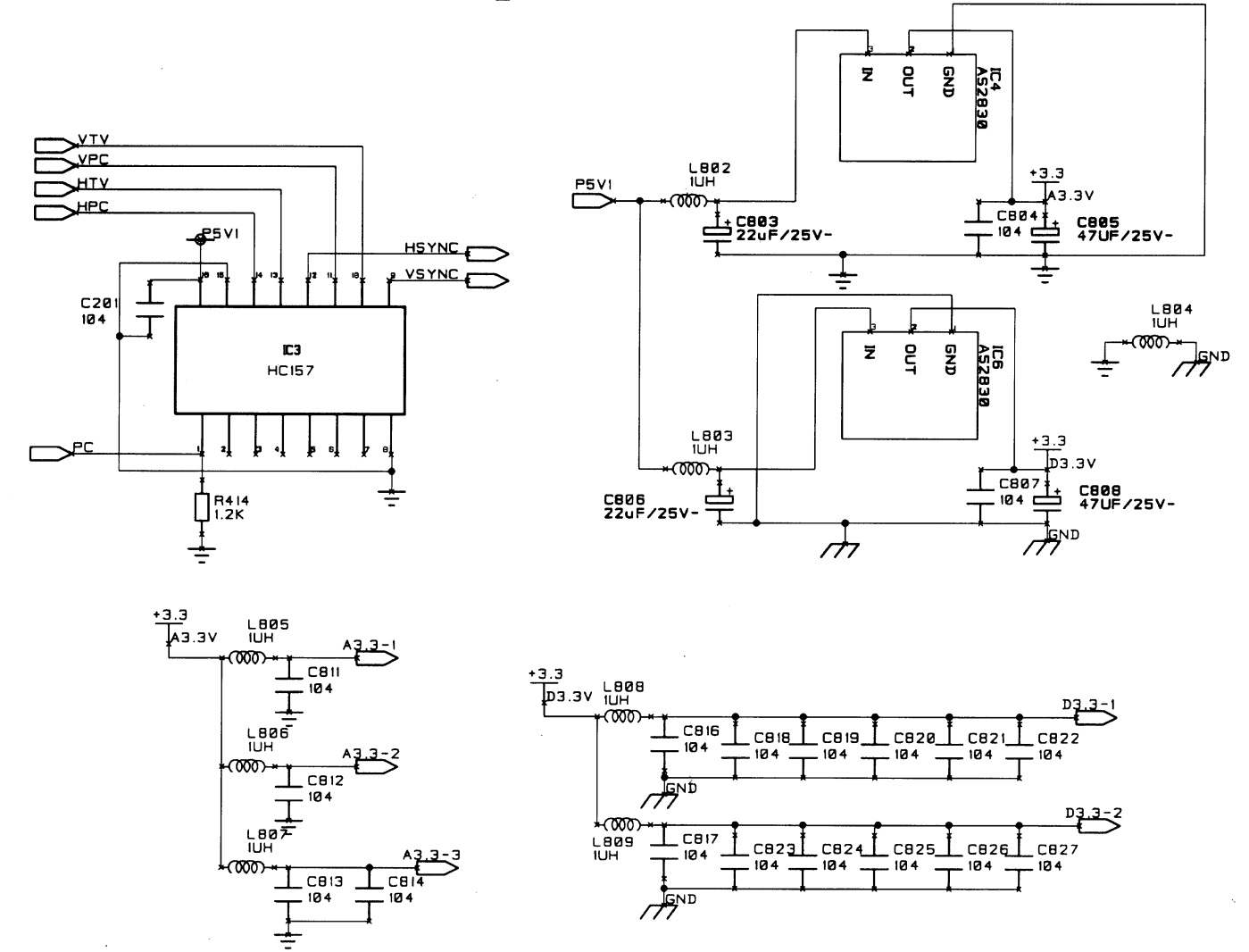
海信牌TDF2901型彩色电视接收机电路图（A2解码板）第2页（共4页）
