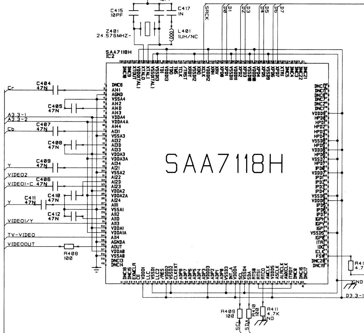
海信牌TDF2901型彩色电视接收机电路图（A2解码板）第2页（共4页）
