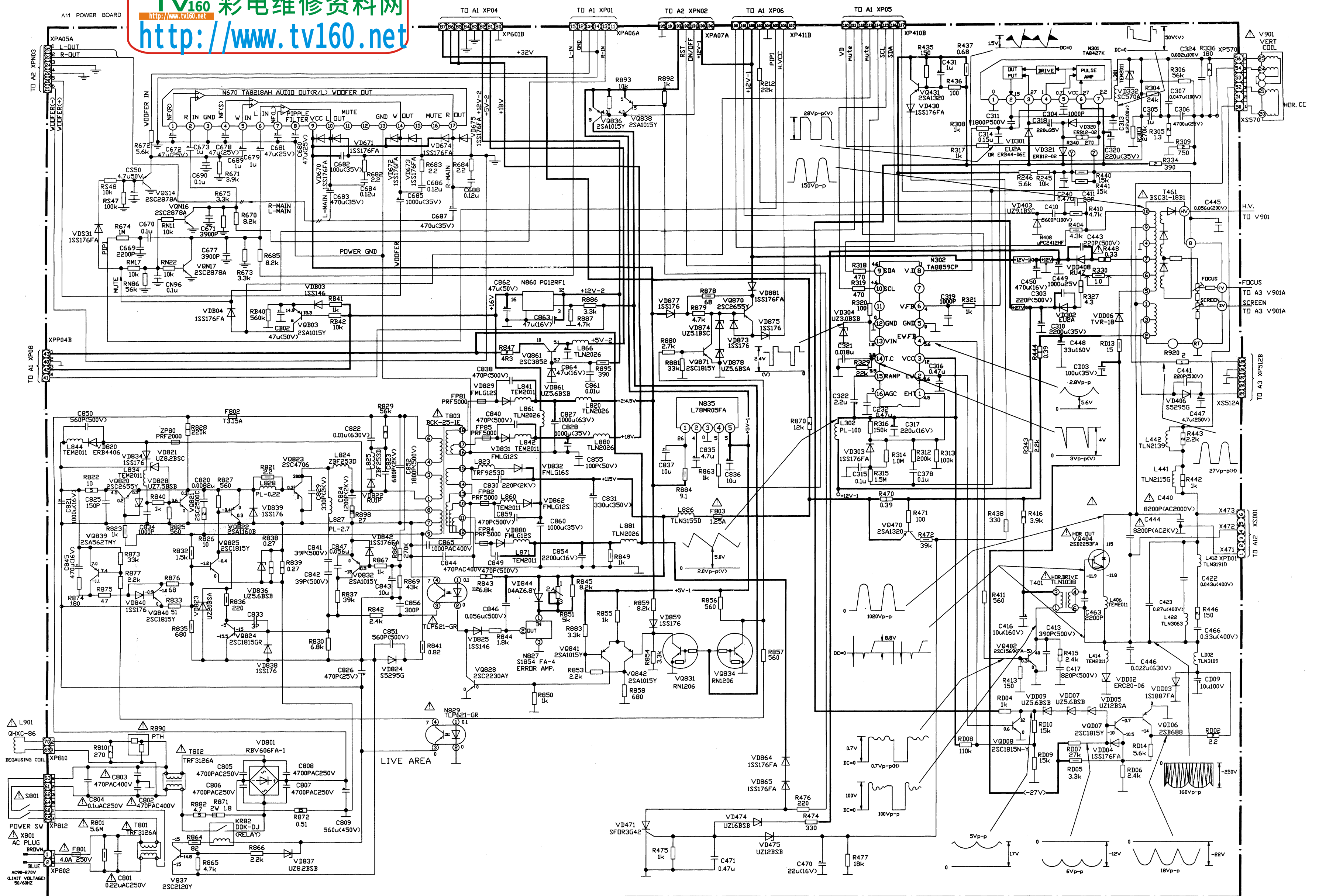
海信牌 TF3430DP 型彩色电视机电路图 (3/4)
