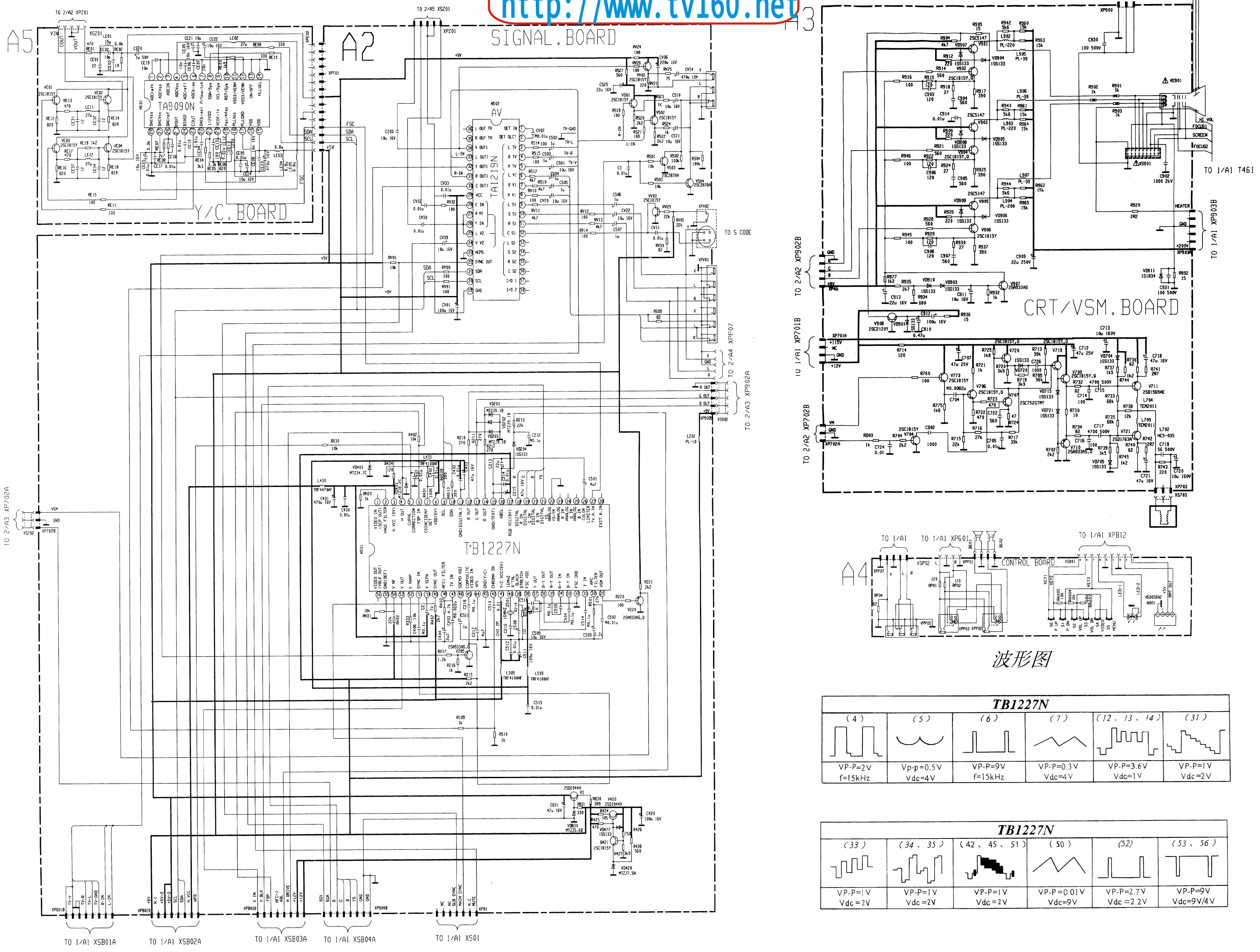
海信牌 TF3400D 型彩色电视机电路图 (A2、A3、A4、A5 板)
