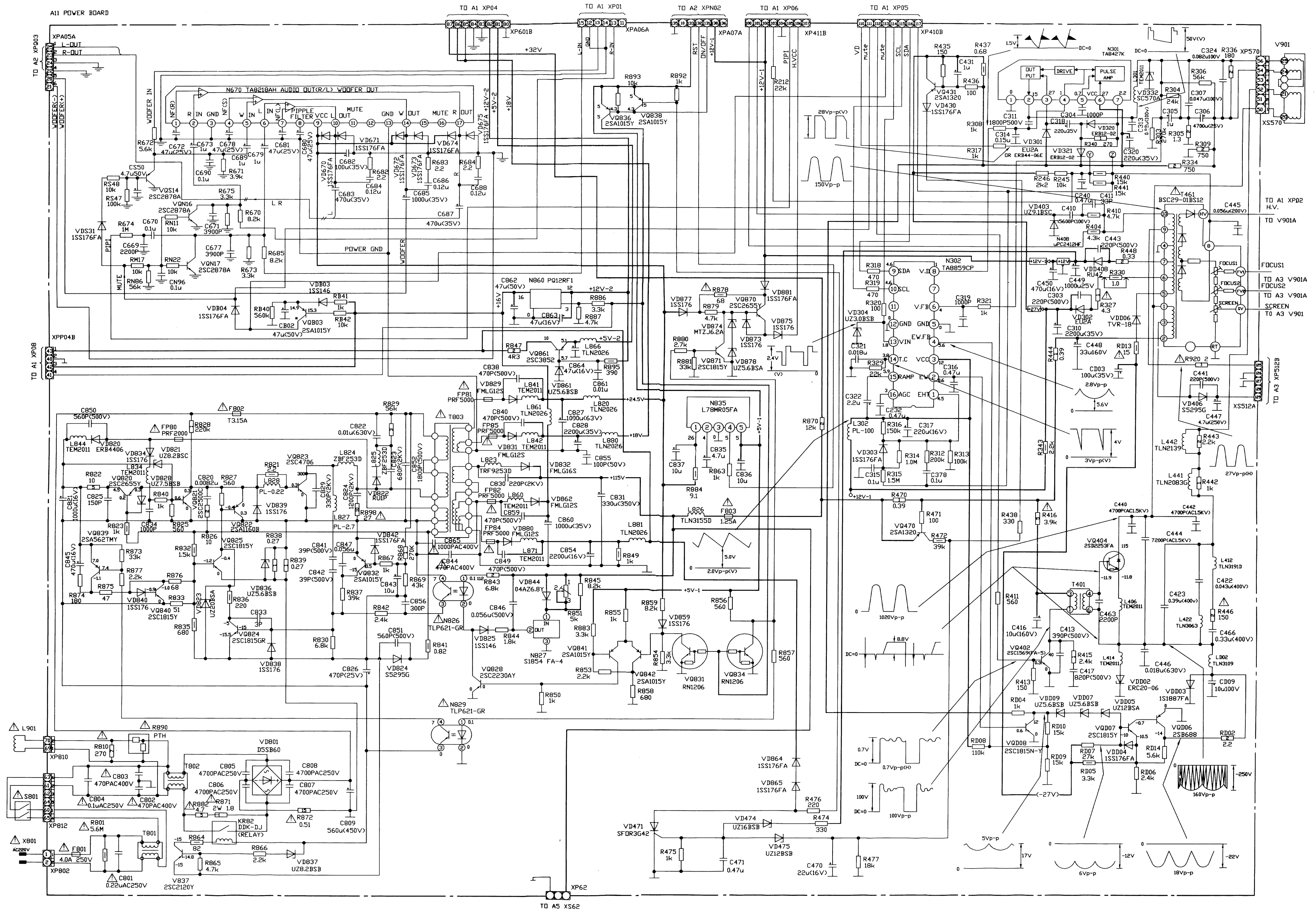
海信牌TF2911FM 型彩色电视机电路图 (3/4)
