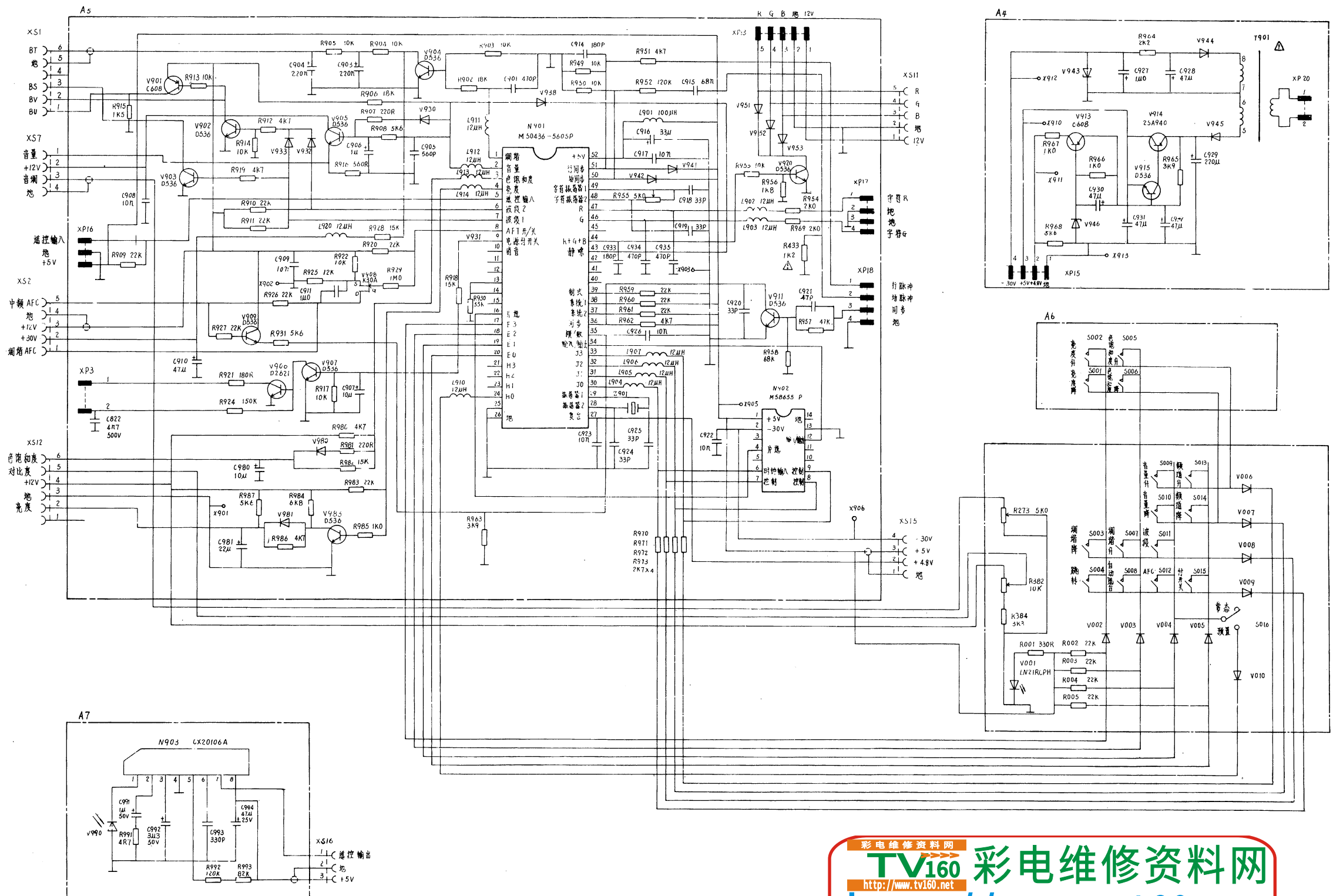
SR5417型彩色电视接收机电路图（遥控线路）
