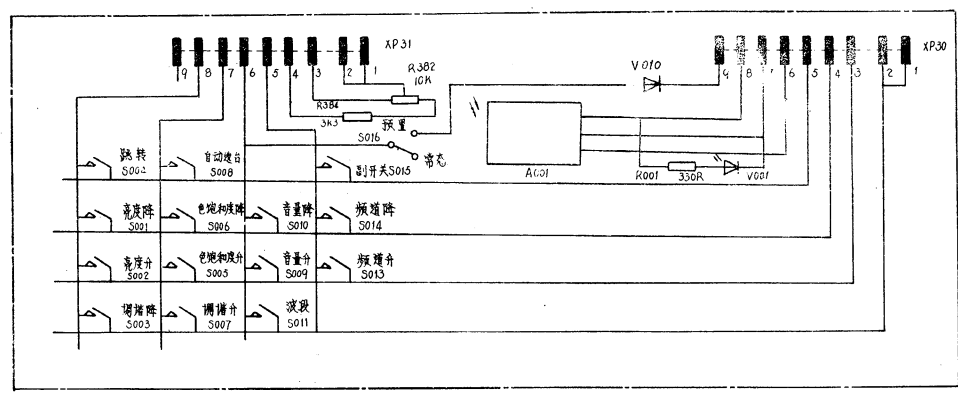
SR4426型彩色电视接收机电路图（遥控线路）
