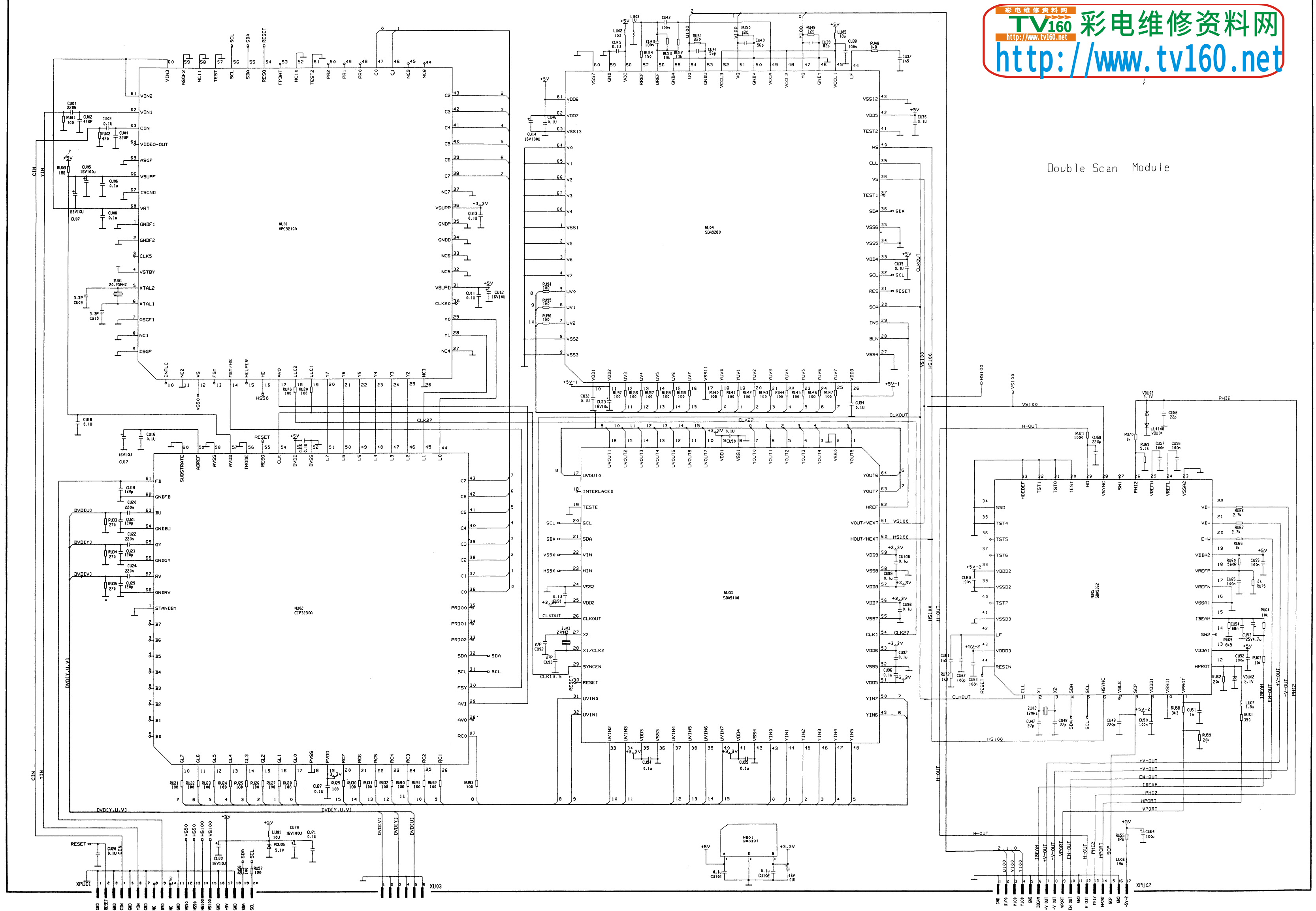
海信牌 TDF29001-3D型彩色电视机电路图 (A4板) 第4页
