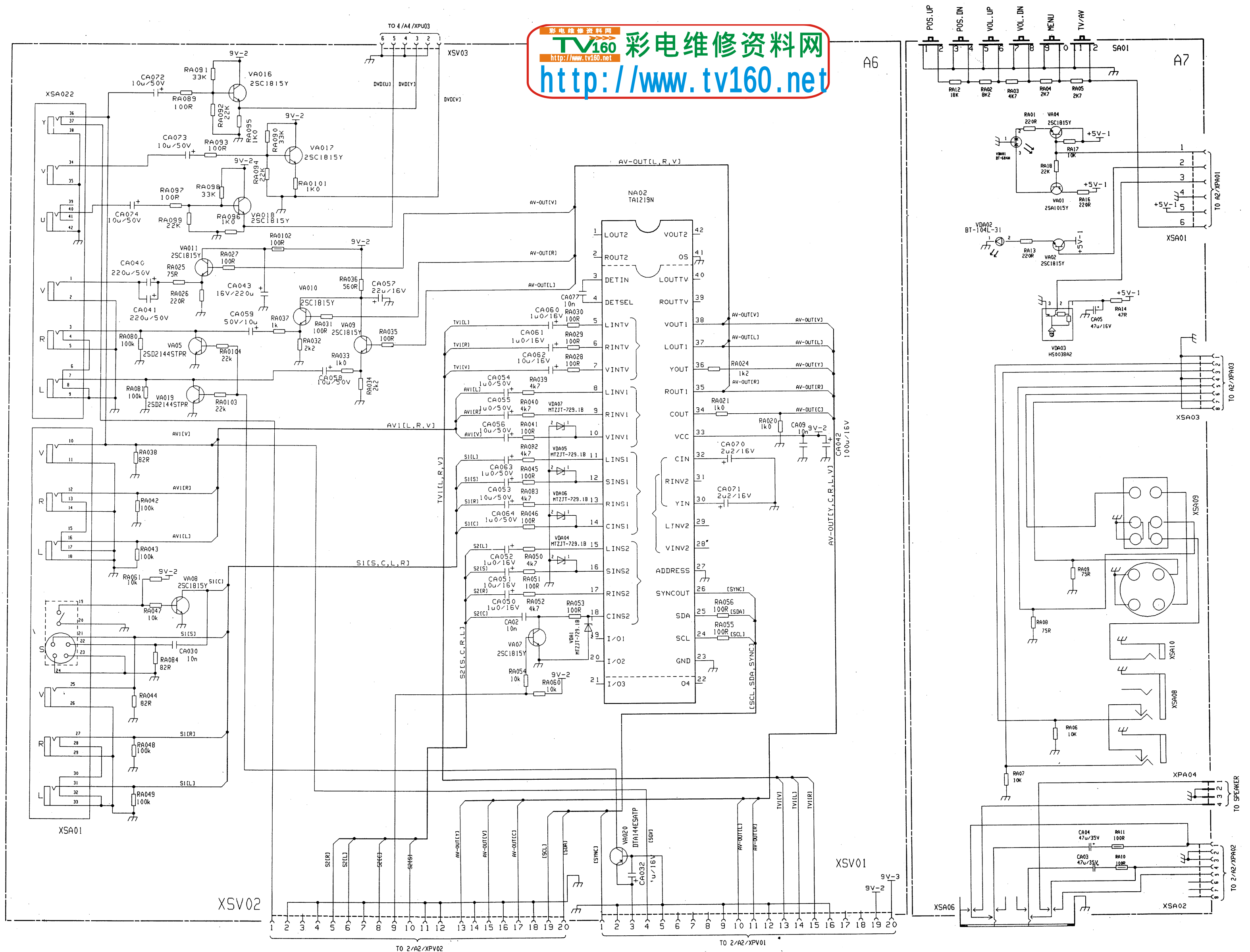
海信牌TDF2918型彩色电视机电路图(A6、A7板)第6页
