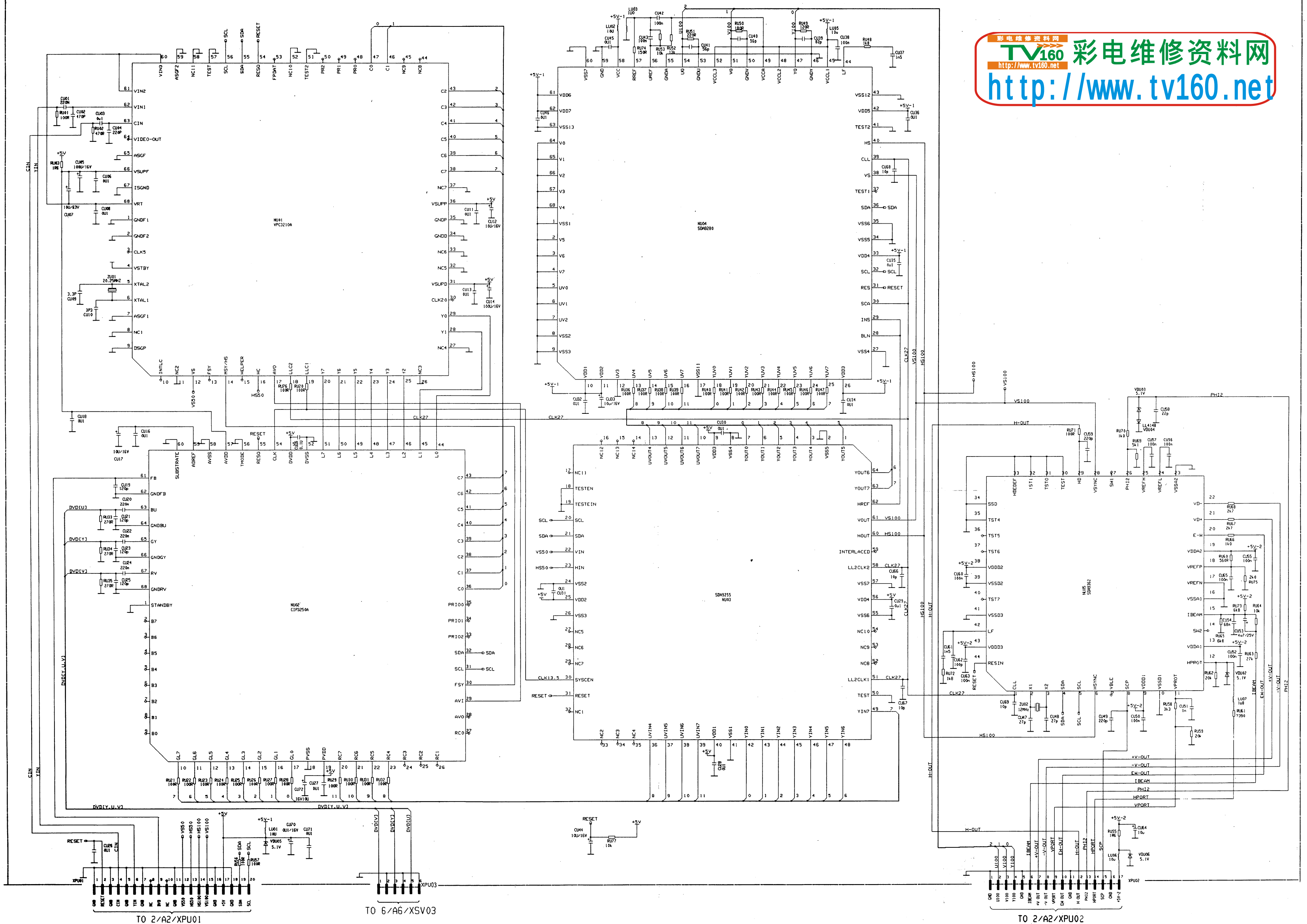
海信牌TDF2918型彩色电视机电路图(A4板) 第4页
