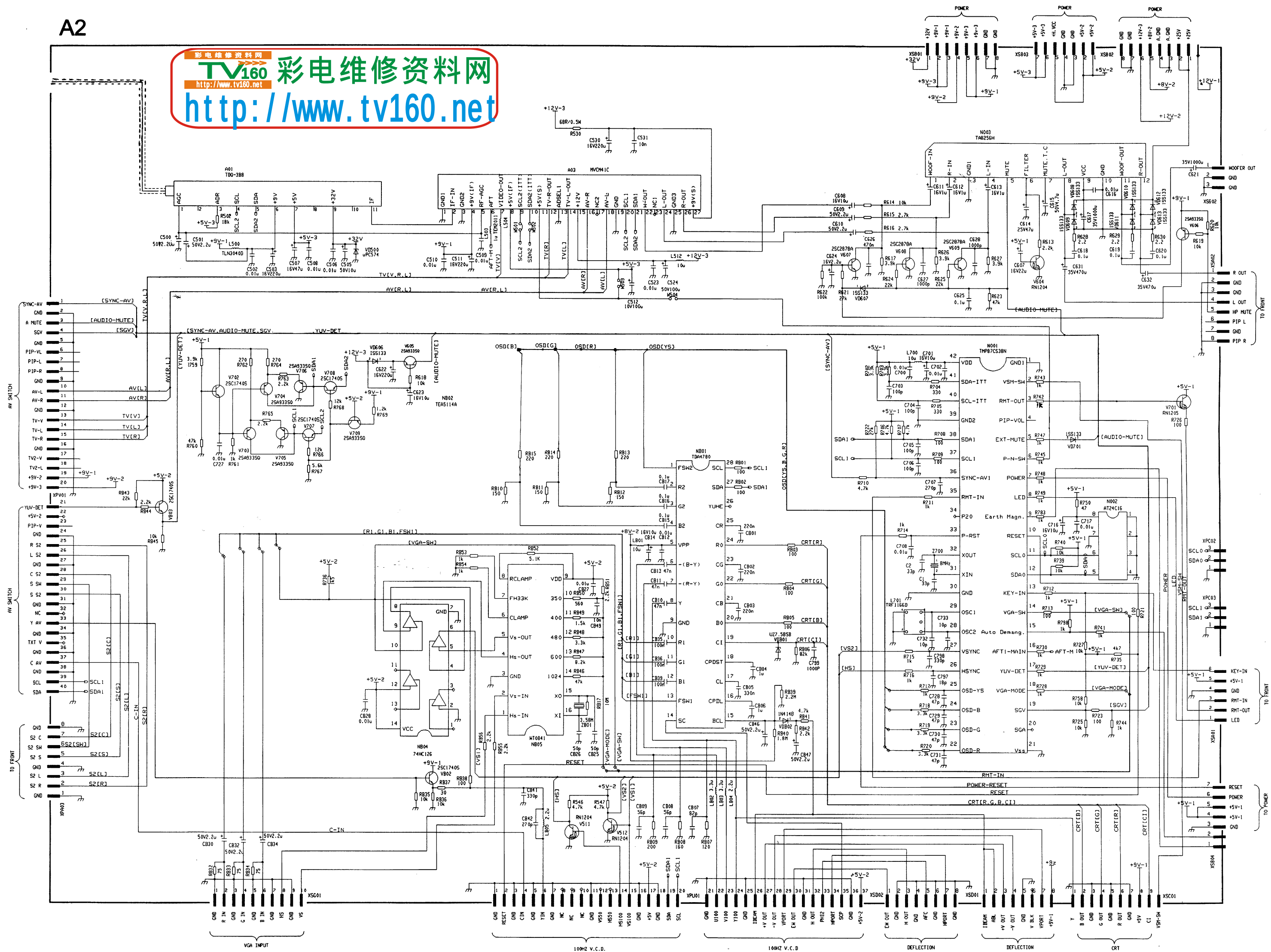
海信牌 TDF2900型彩色电视机电路图 (A2板) 共6页 第2页
