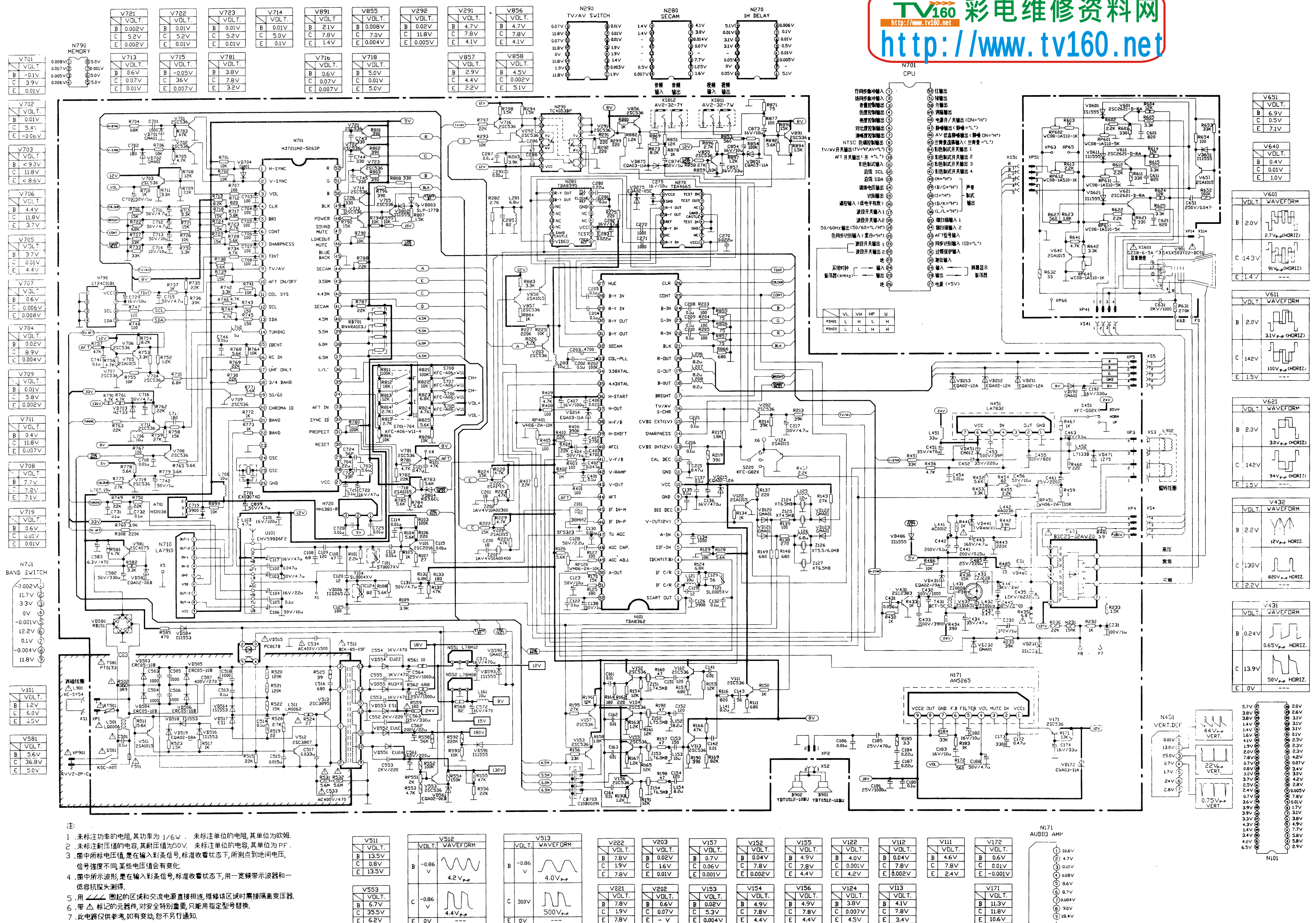
TC2127FA/TC2128FA型彩色电视接收机电路图
