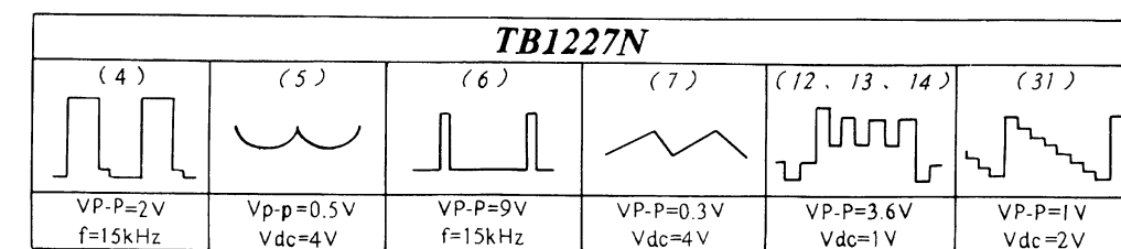
波形图
