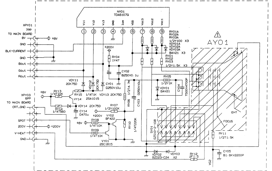
Y Board JU7. 820. 1586
