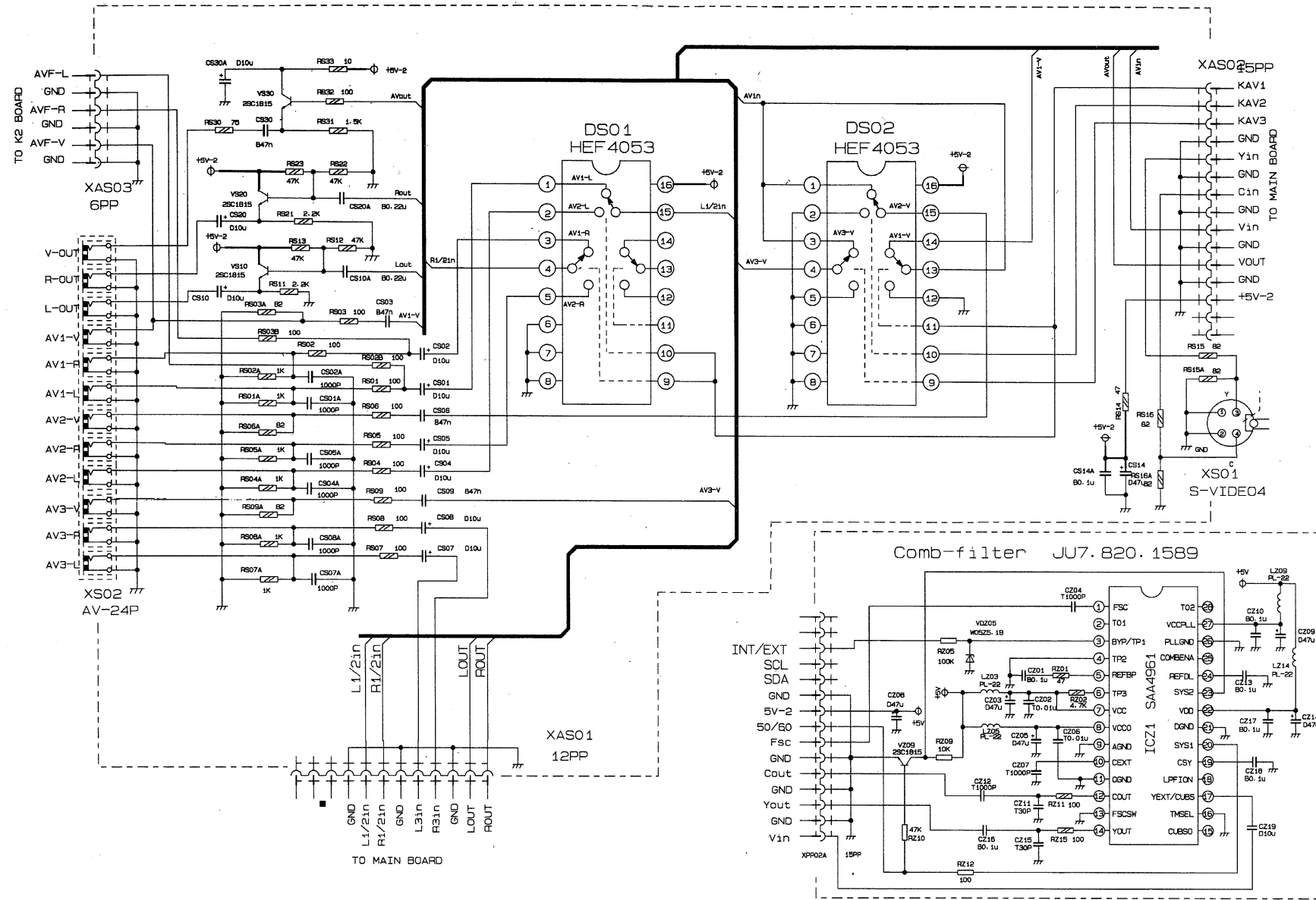
AV BOARD JU7.820.1585-2
