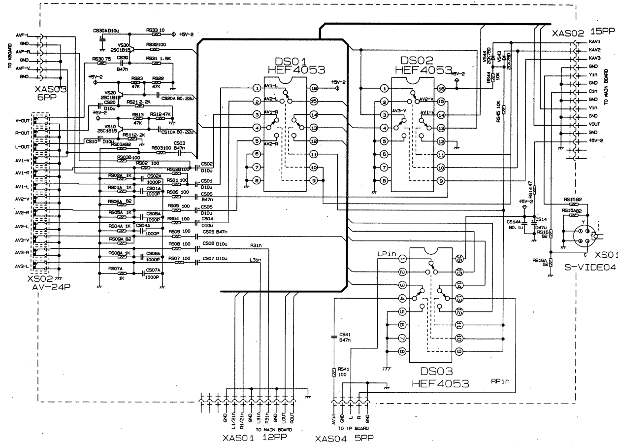
AV Board JU7.820.1585-1
