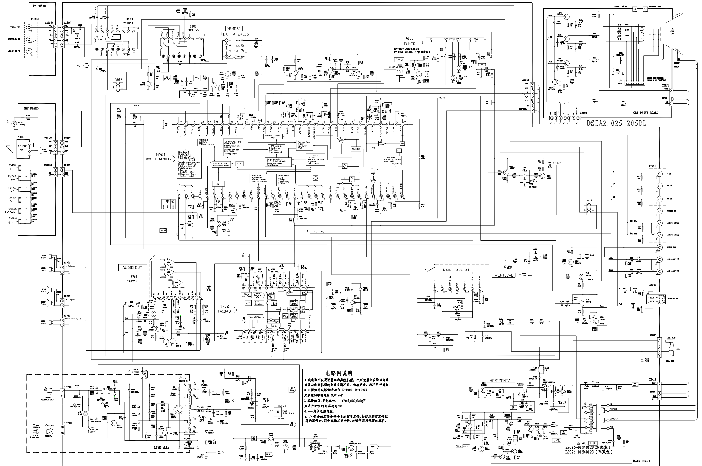
创佳牌 (CJ20机芯) 大屏幕彩色电视机电原理图
