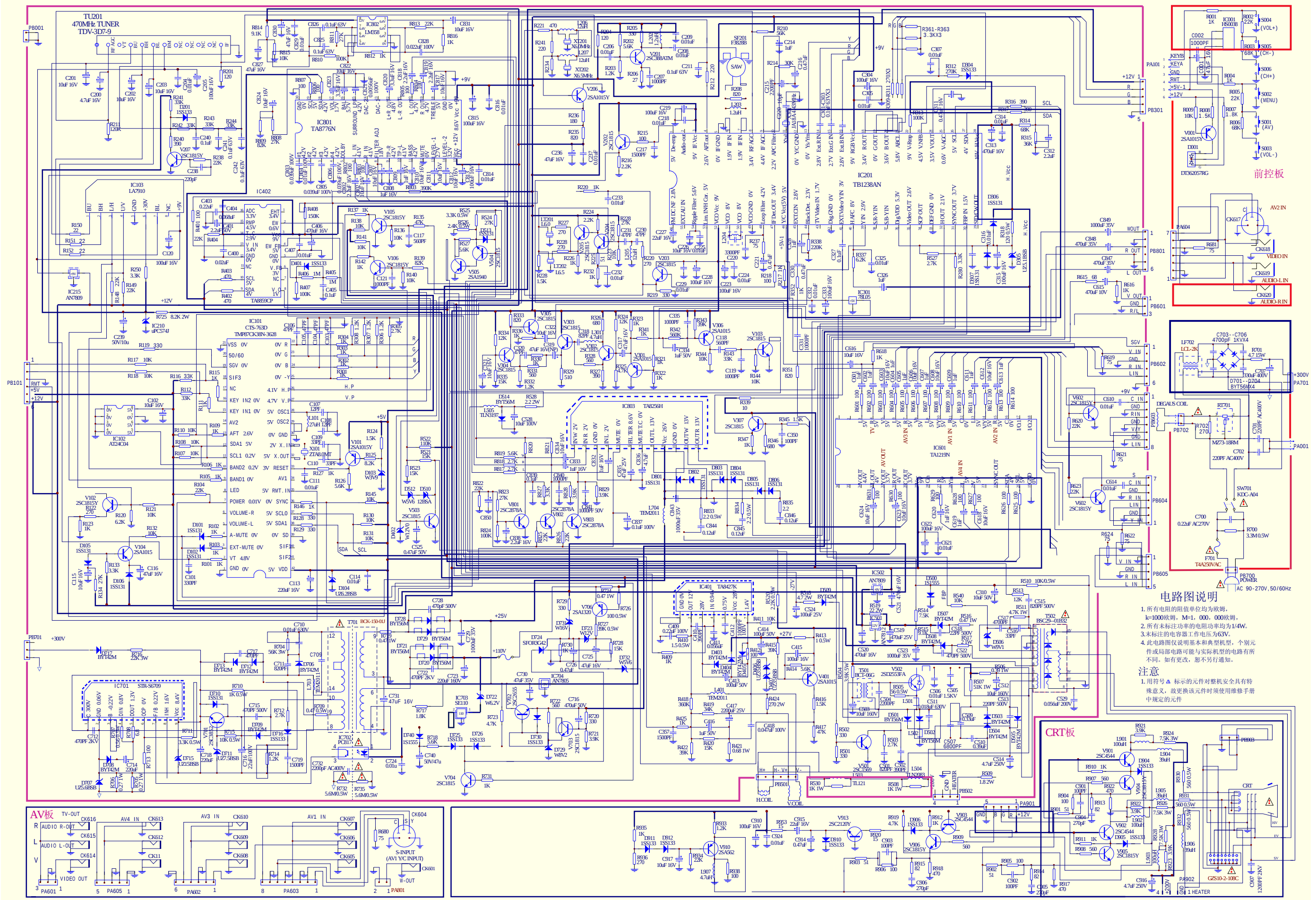
创佳牌 LT系列大屏幕彩色电视机电原理图 (CJ13机芯)
