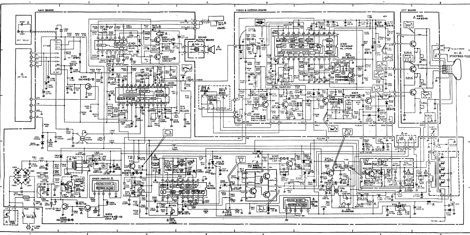
图一 金星牌C37-401彩色电视机原理图(HAM)
